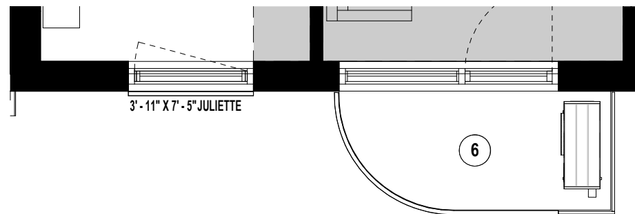
EXTRAIT FENÊTRE DE L'UNITÉ 1802
