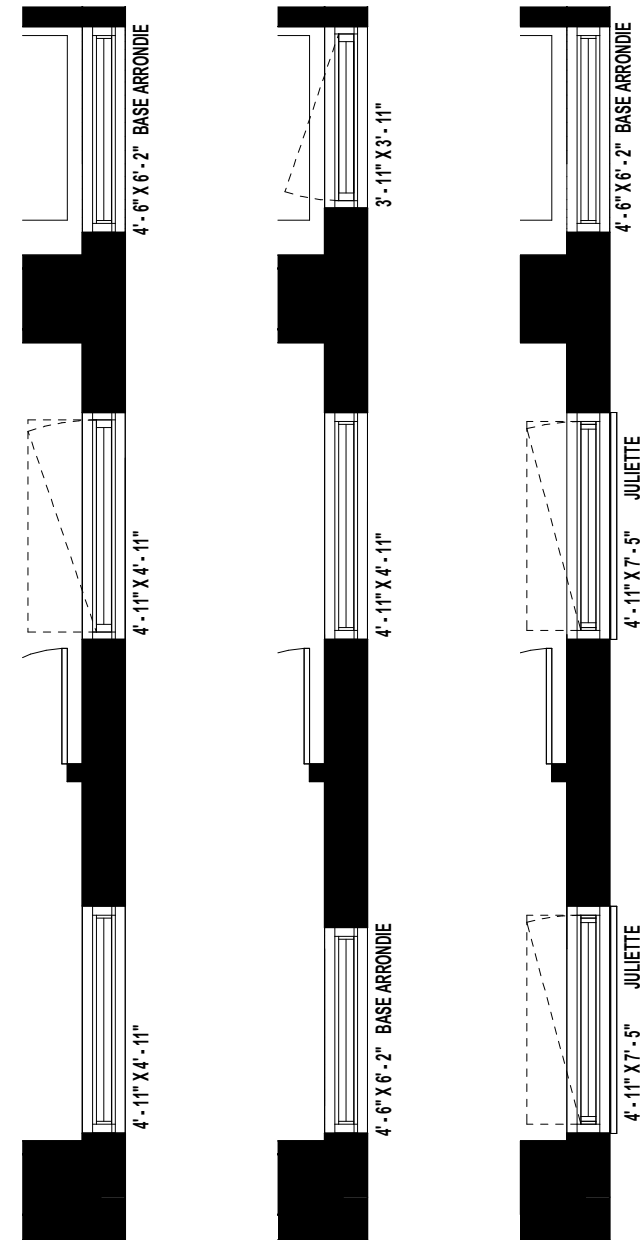
EXTRAIT FENÊTRE DE L'UNITÉ 919
